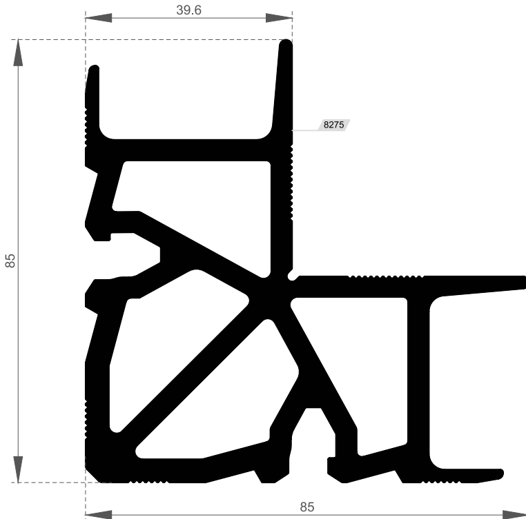
OM-5114 Köşe Takoz Profili / Corner Cleat Profile
