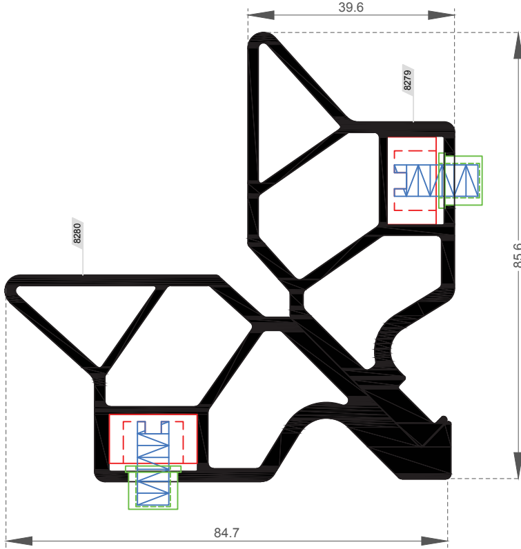
OM-5144 Köşe Takoz Profili / Corner Cleat Profile
